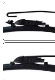
Крепление «Крючок»
